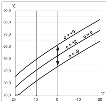
Коррекция кривой нагрева для C=12
