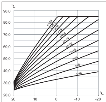
Коэффициент наклона кривой нагрева
